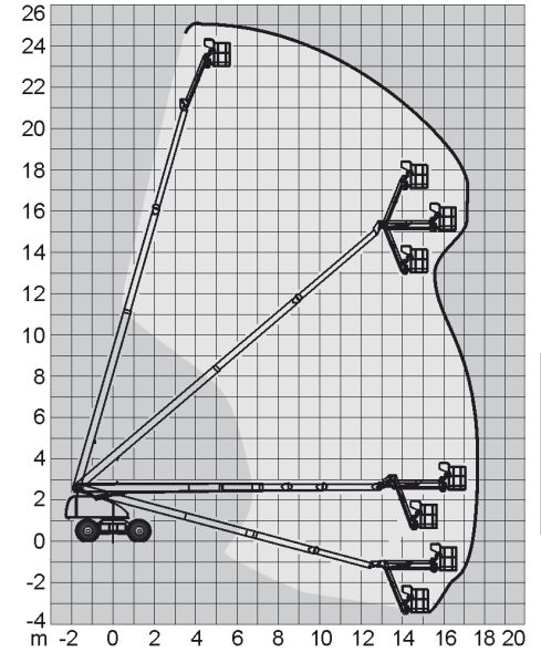
F-25 TKX
